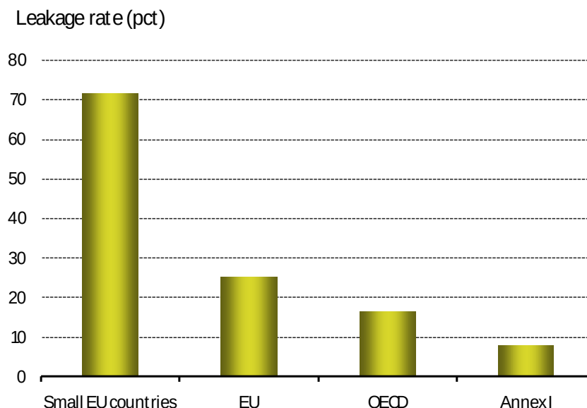
Figur: Koldioxidläckage beroende på regionens storlek
